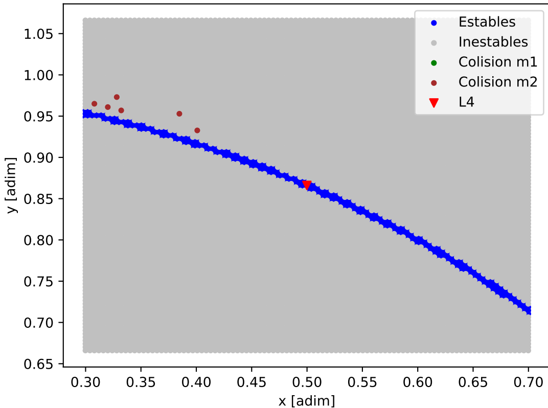
Mapa de estabilidad - KOI-134
