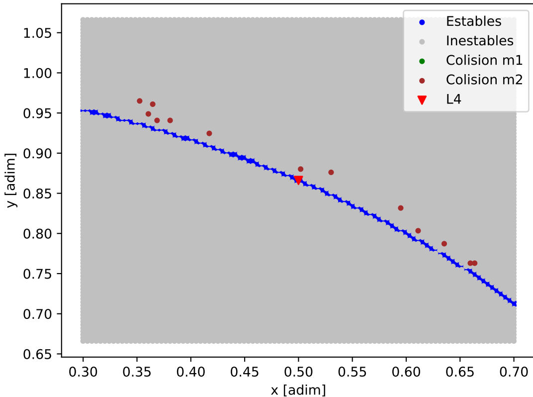
Mapa de estabilidad - TOI-5126
