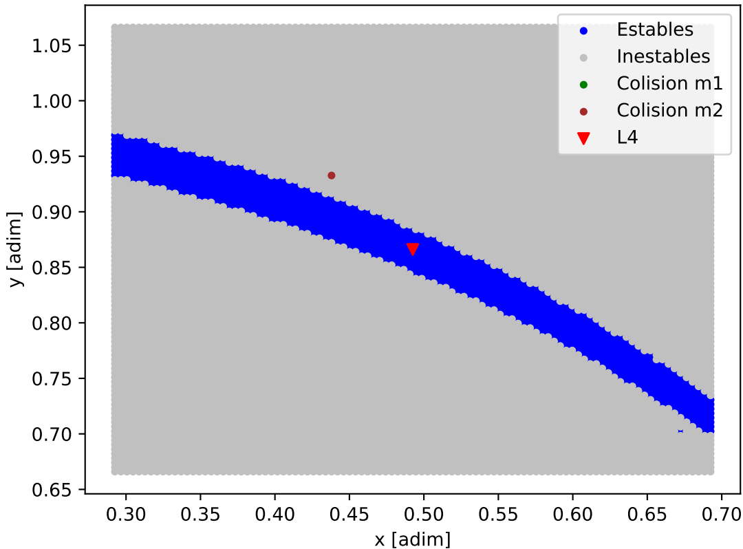
Mapa de estabilidad - ups_And
