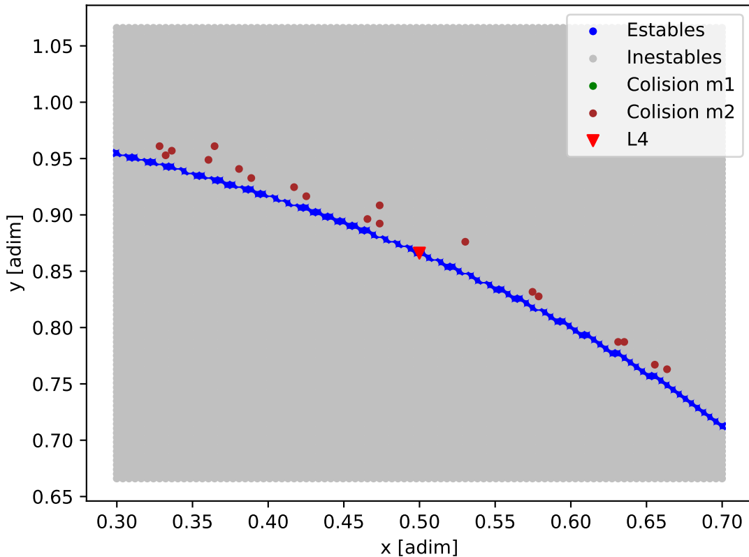
Mapa de estabilidad - 61_Vir
