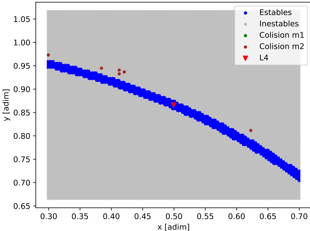
Mapa de estabilidad - HAT-P-13
