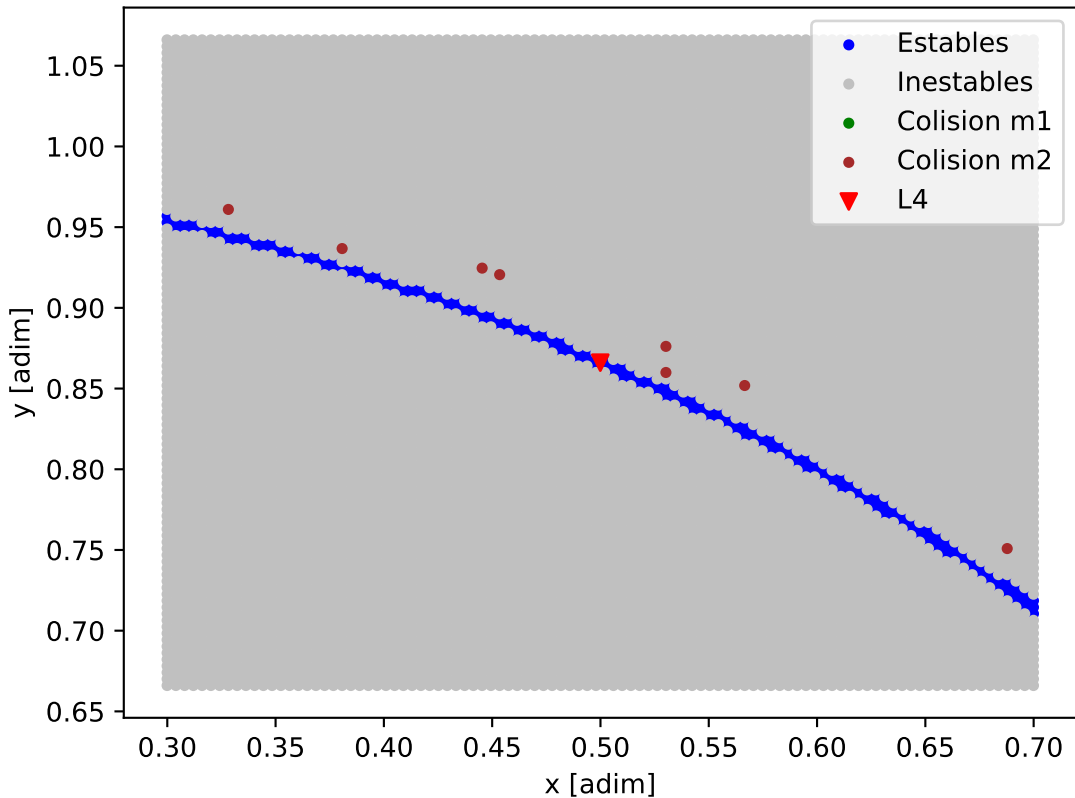
Mapa de estabilidad - HD_11964
