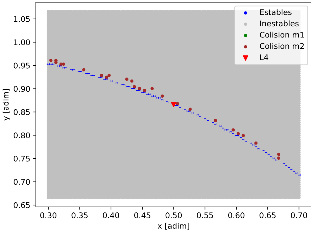
Mapa de estabilidad - HD_134606
