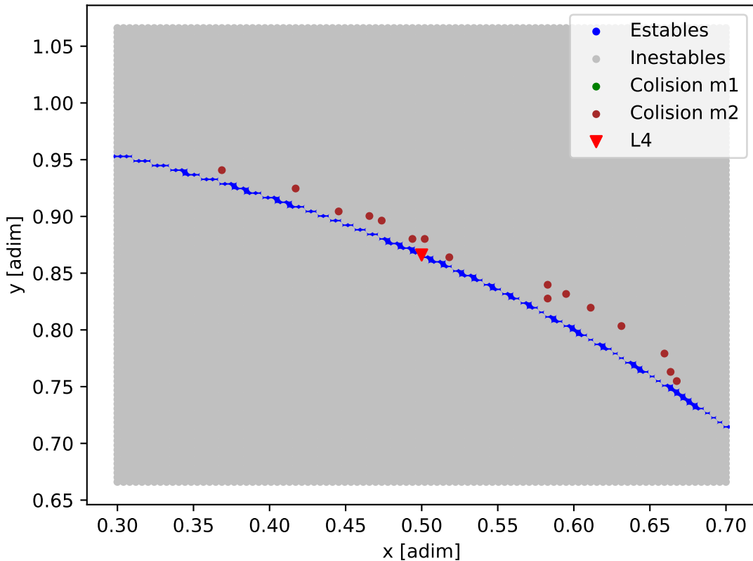
Mapa de estabilidad - HD_136352
