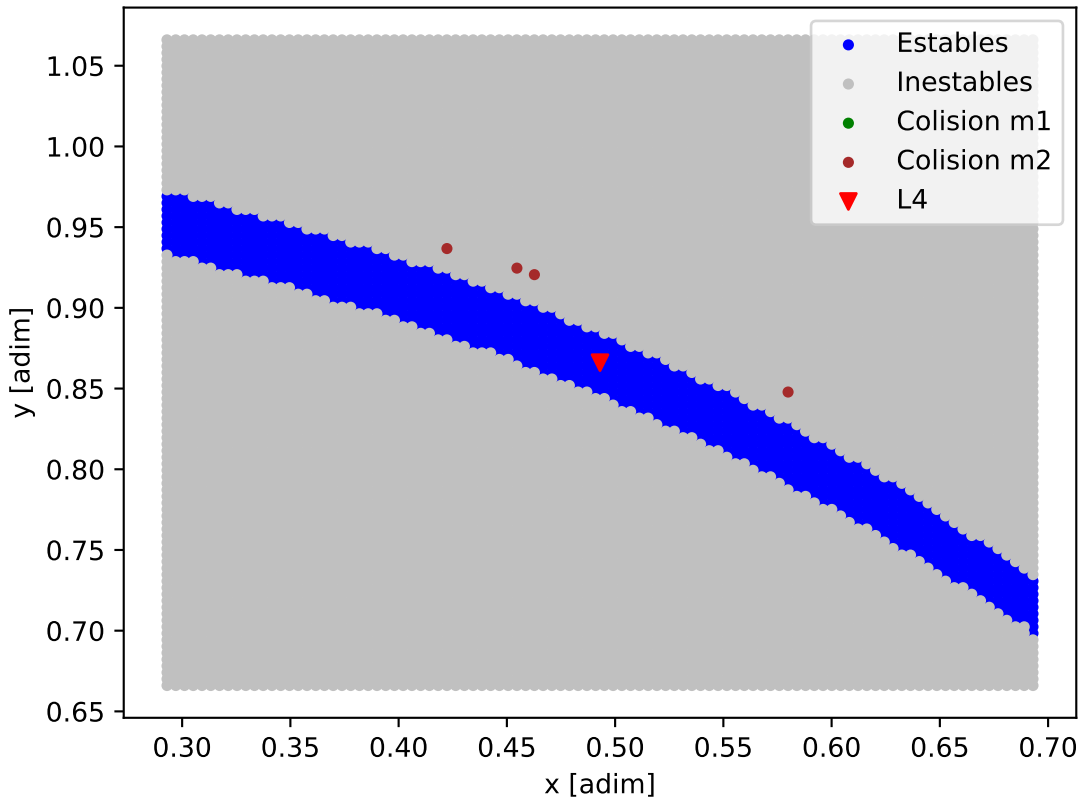
Mapa de estabilidad - HD_137496
