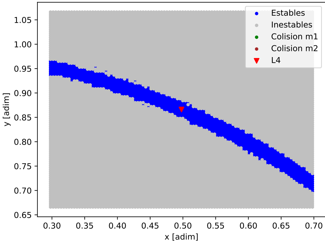
Mapa de estabilidad - HD_147018
