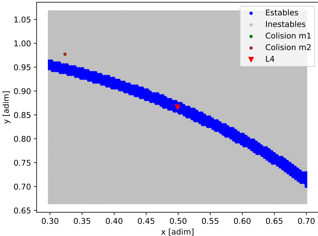
Mapa de estabilidad - HD_159243
