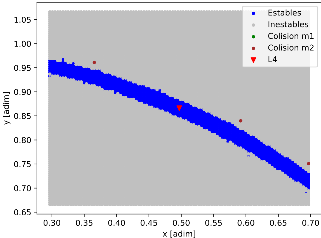
Mapa de estabilidad - HD_183263
