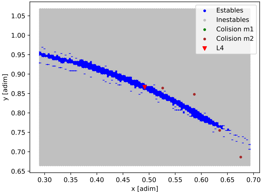
Mapa de estabilidad - HD_183263
