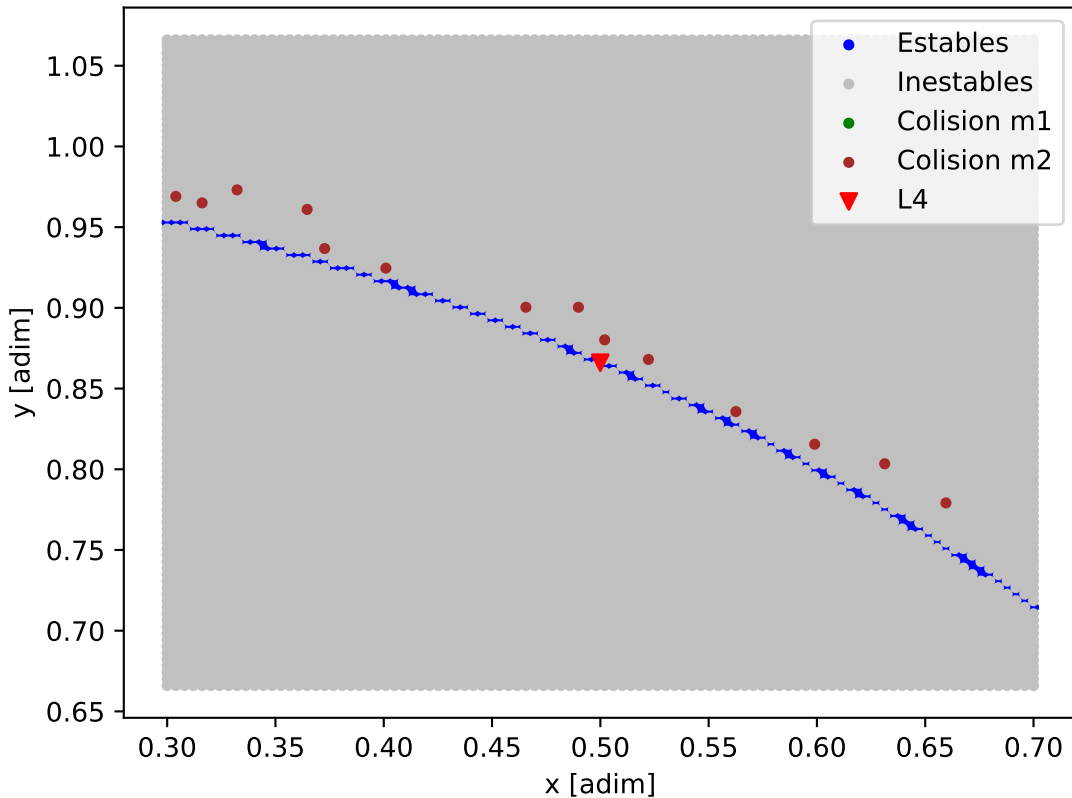
Mapa de estabilidad - HD_189567
