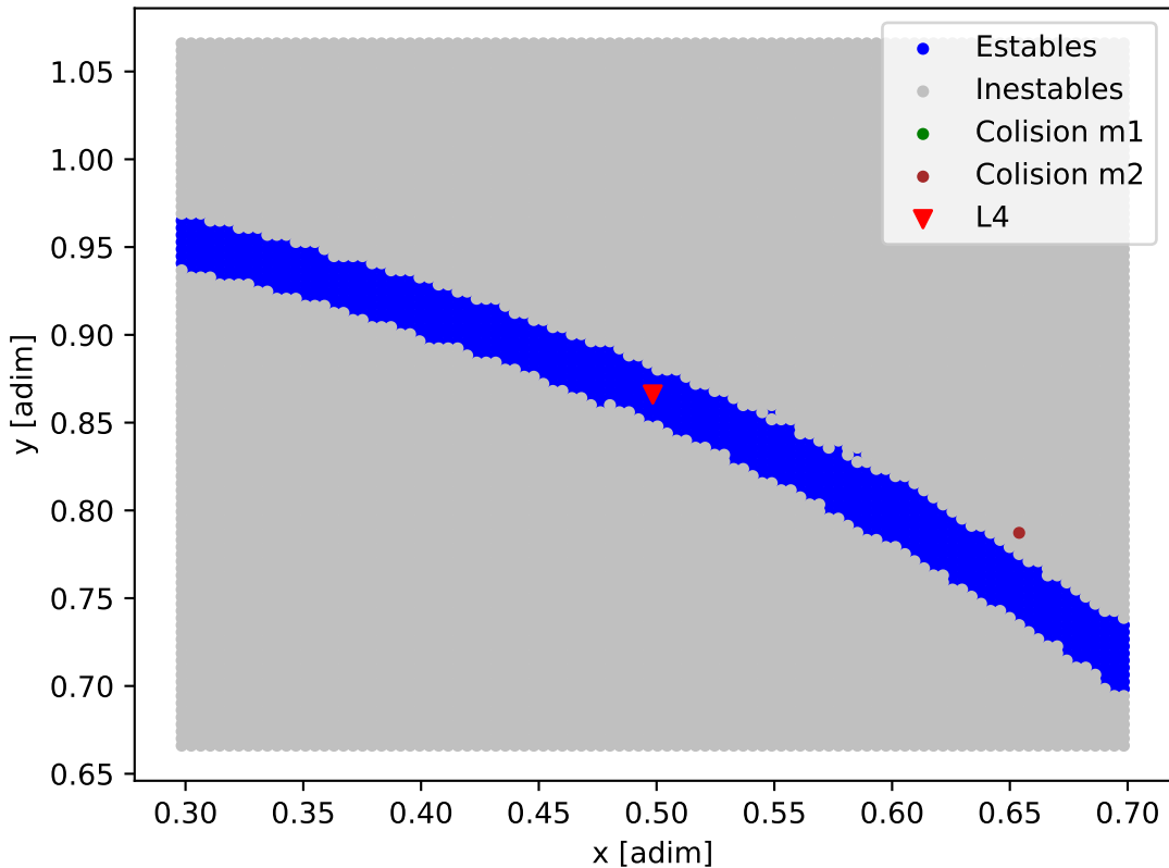
Mapa de estabilidad - HD_190360
