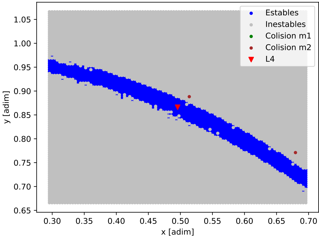
Mapa de estabilidad - HD_24040
