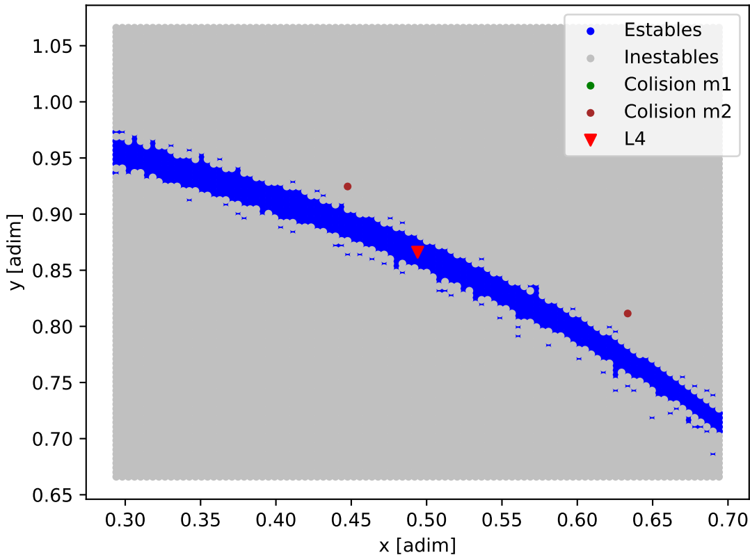
Mapa de estabilidad - HD_30177
