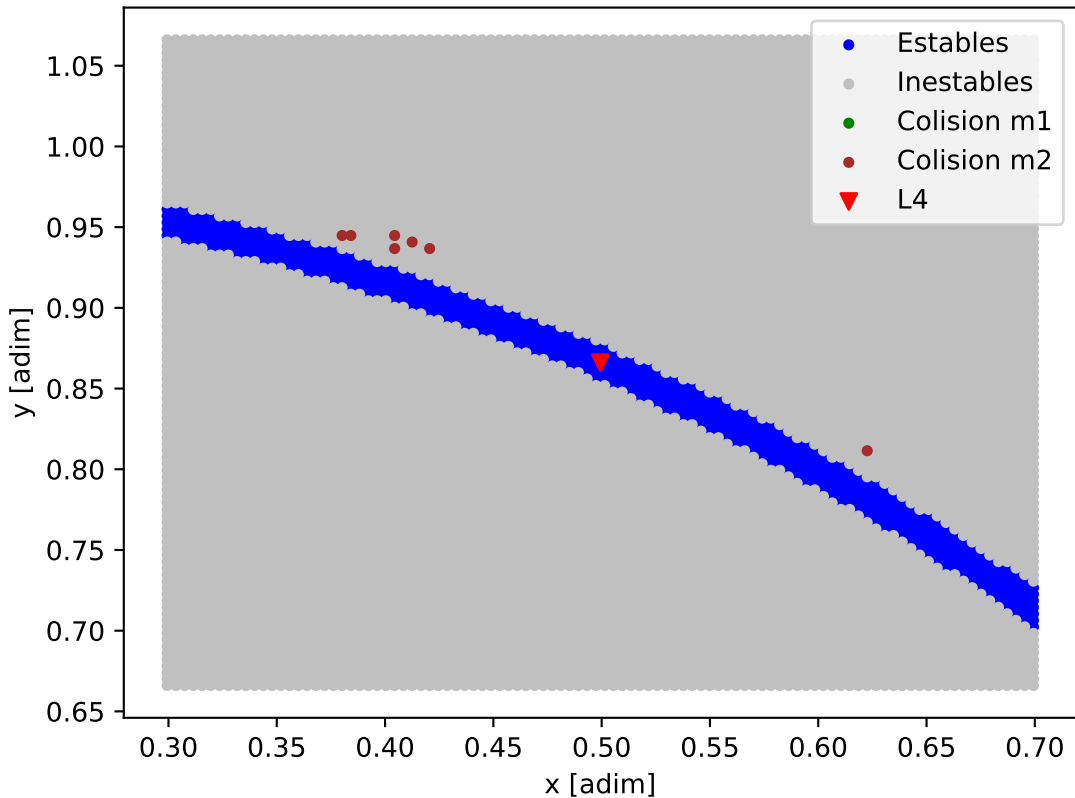
Mapa de estabilidad - HD_38529
