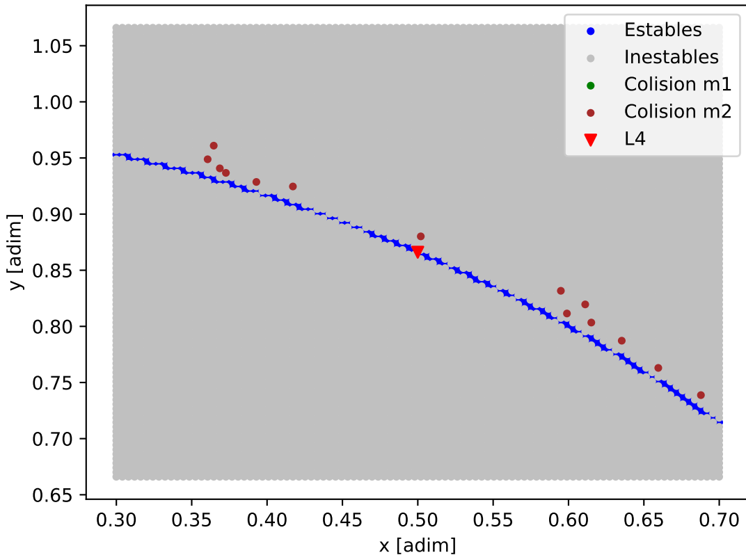
Mapa de estabilidad - HD_39091
