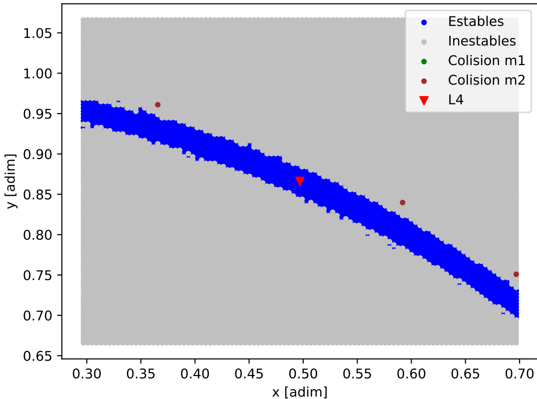
Mapa de estabilidad - HD_48265
