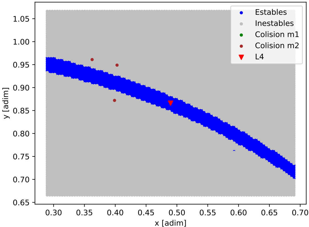
Mapa de estabilidad - HD_66428
