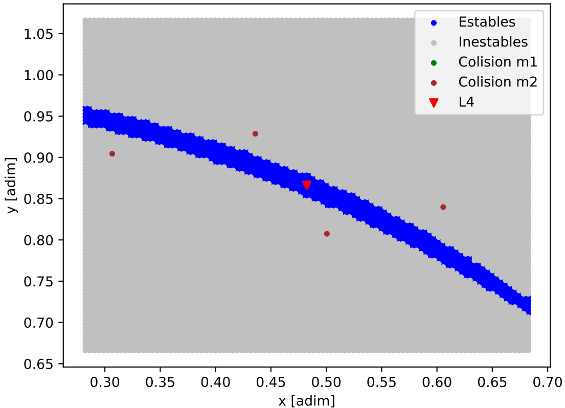
Mapa de estabilidad - HD_72659
