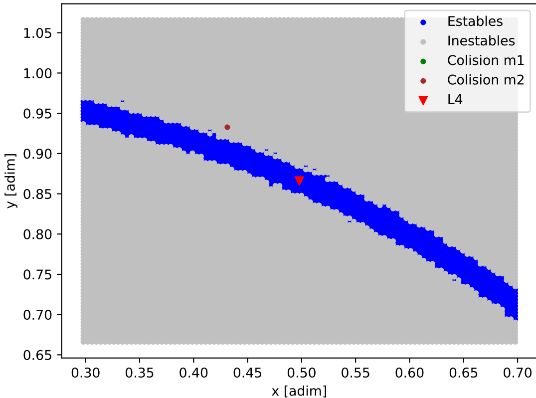
Mapa de estabilidad - HD_73526
