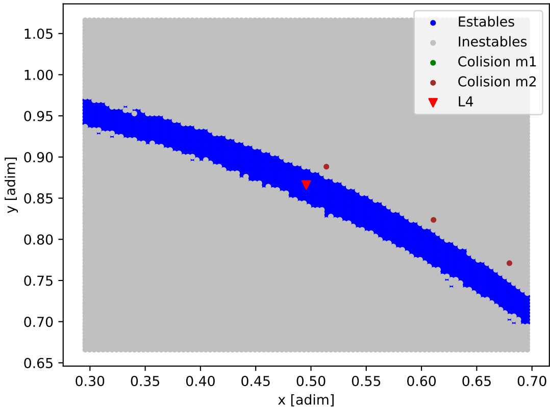
Mapa de estabilidad - HD_75784
