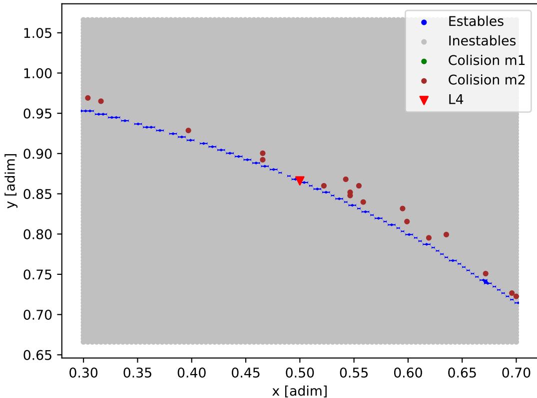
Mapa de estabilidad - HD_80653
