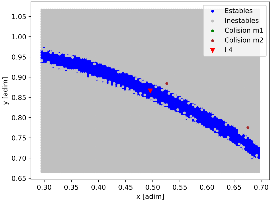
Mapa de estabilidad - HD_80653
