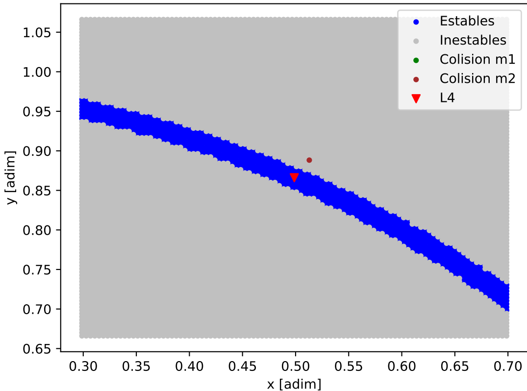
Mapa de estabilidad - HIP_14810
