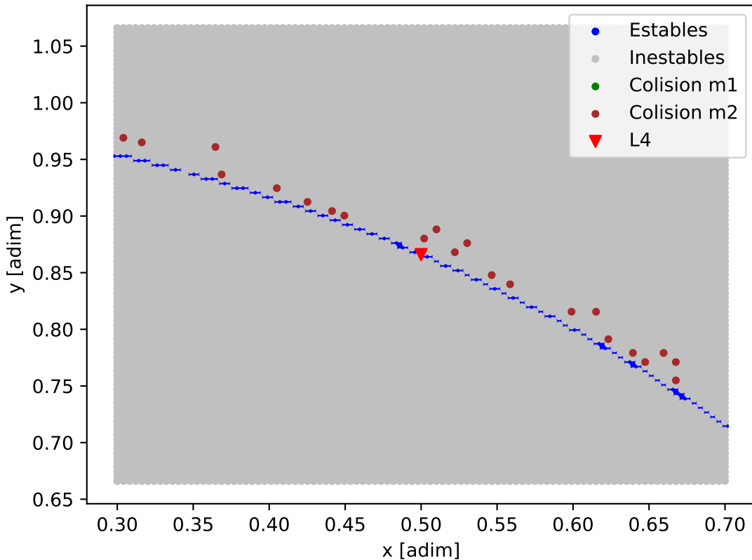
Mapa de estabilidad - K2-111
