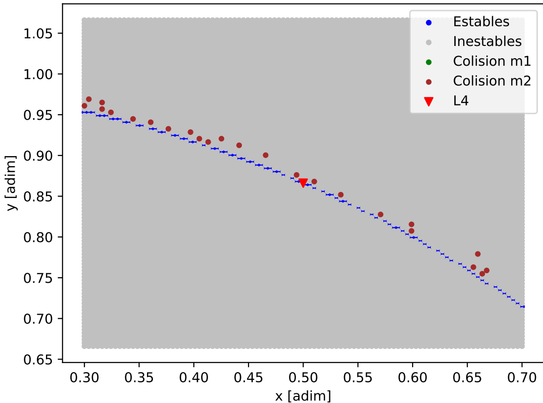
Mapa de estabilidad - K2-37
