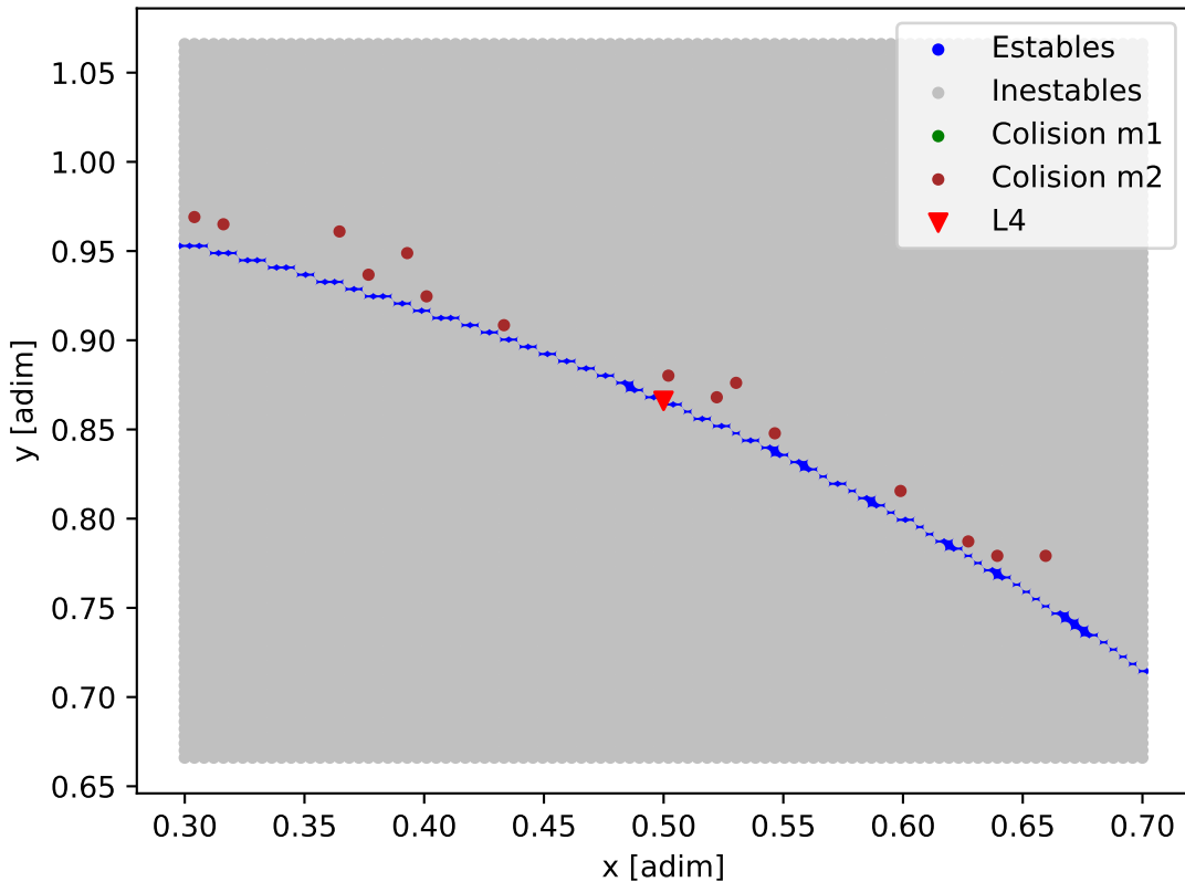
Mapa de estabilidad - K2-38
