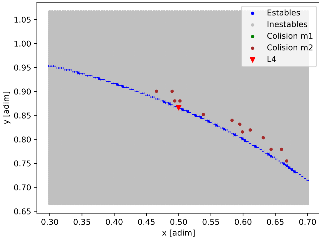
Mapa de estabilidad - Kepler-103
