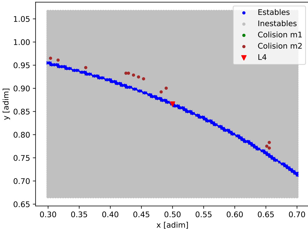
Mapa de estabilidad - Kepler-129
