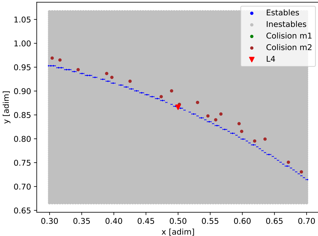
Mapa de estabilidad - Kepler-69
