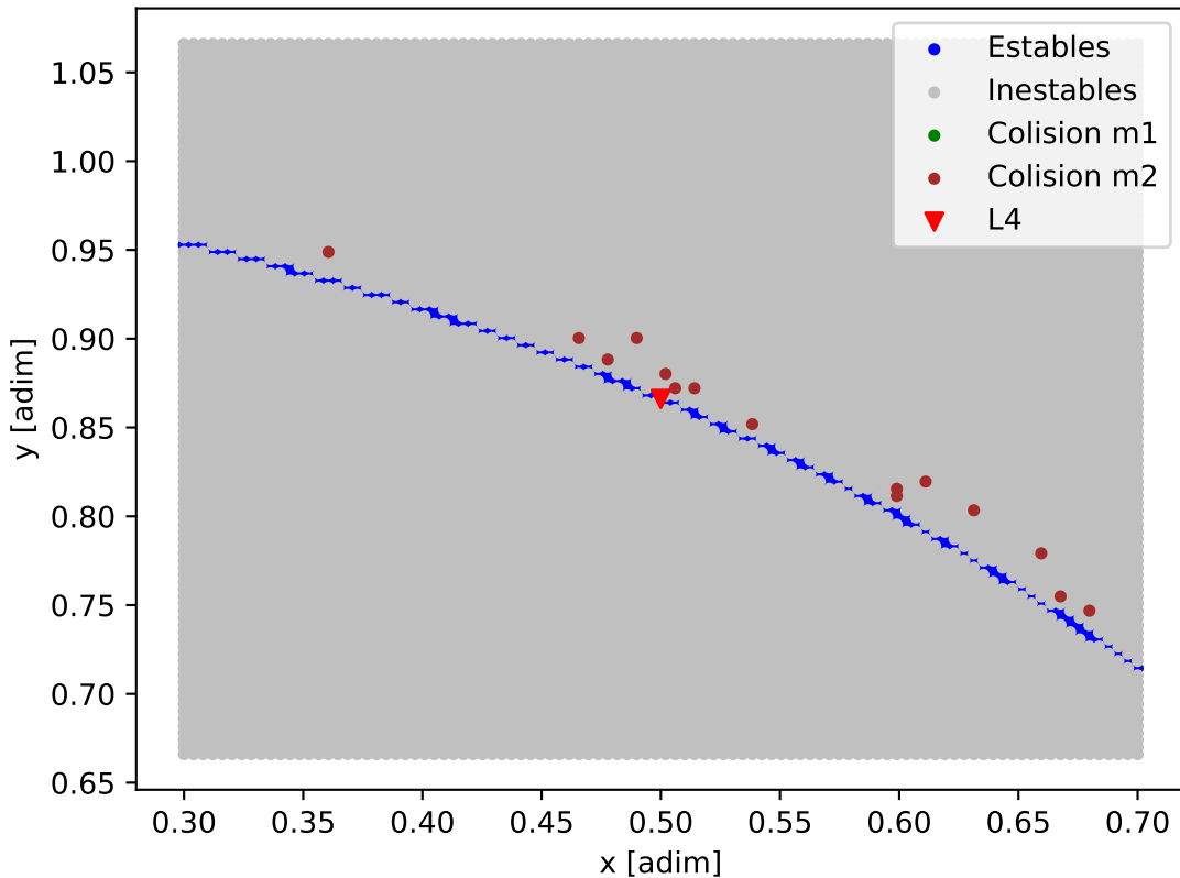
Mapa de estabilidad - Kepler-963
