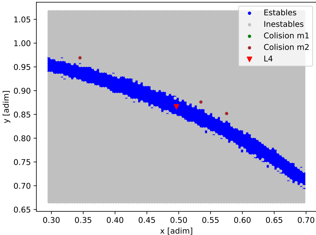
Mapa de estabilidad - OGLE-2019-BLG-0468L
