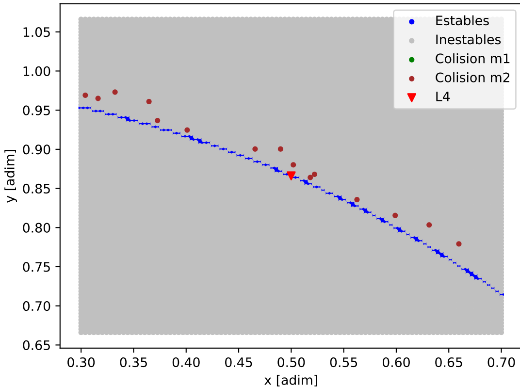
Mapa de estabilidad - TOI-1203
