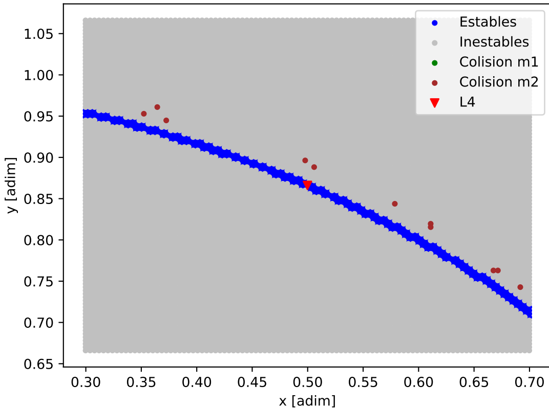
Mapa de estabilidad - TOI-1386
