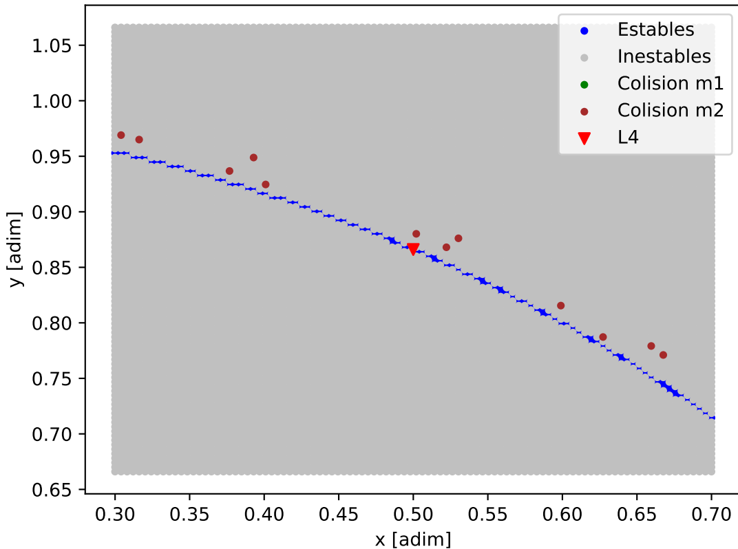
Mapa de estabilidad - TOI-561
