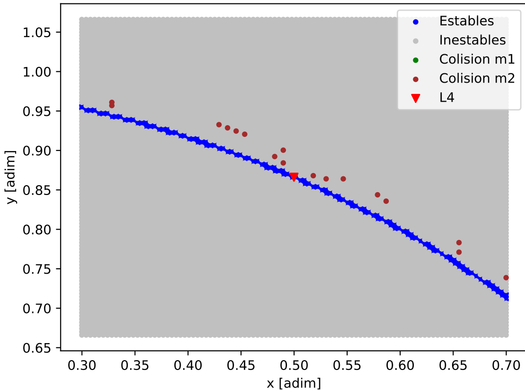
Mapa de estabilidad - TOI-6041
