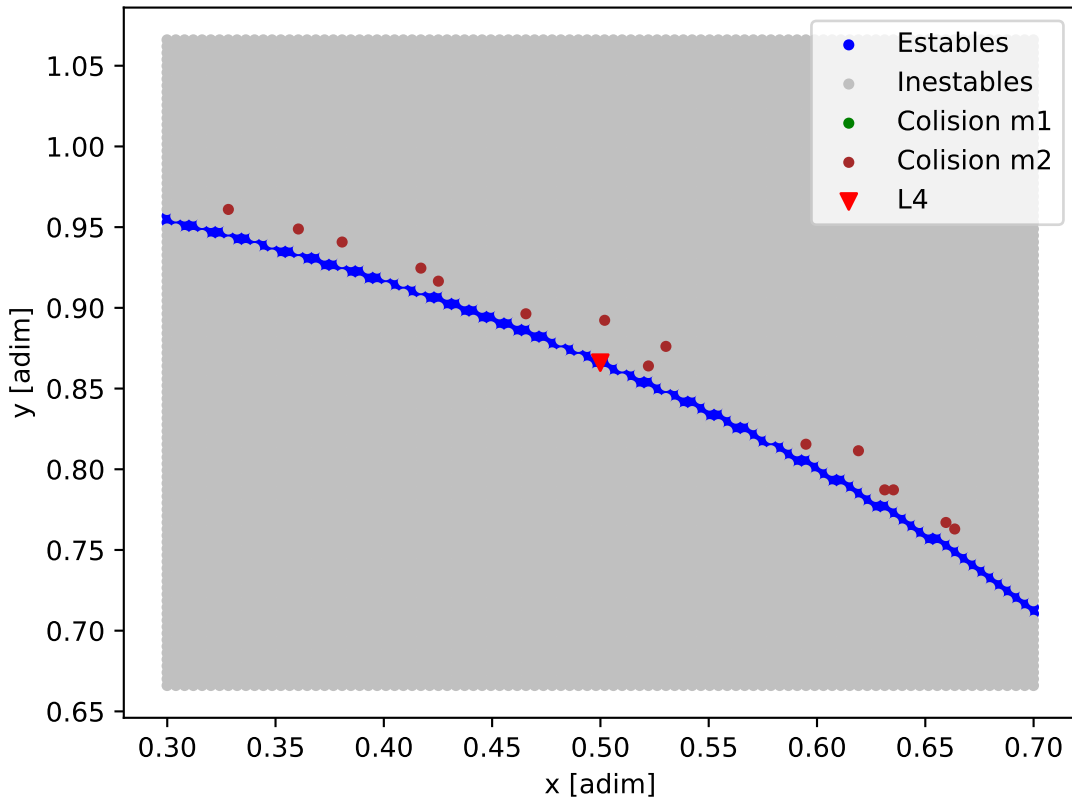
Mapa de estabilidad - TOI-6109
