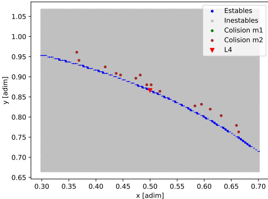
Mapa de estabilidad - TOI-763
