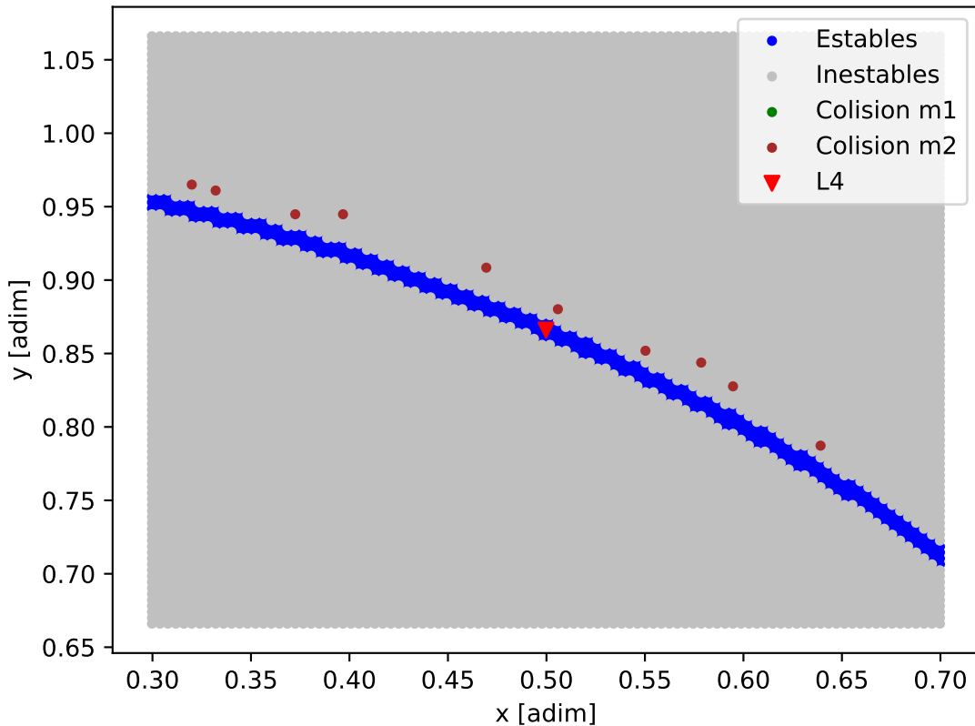
Mapa de estabilidad - WASP-126
