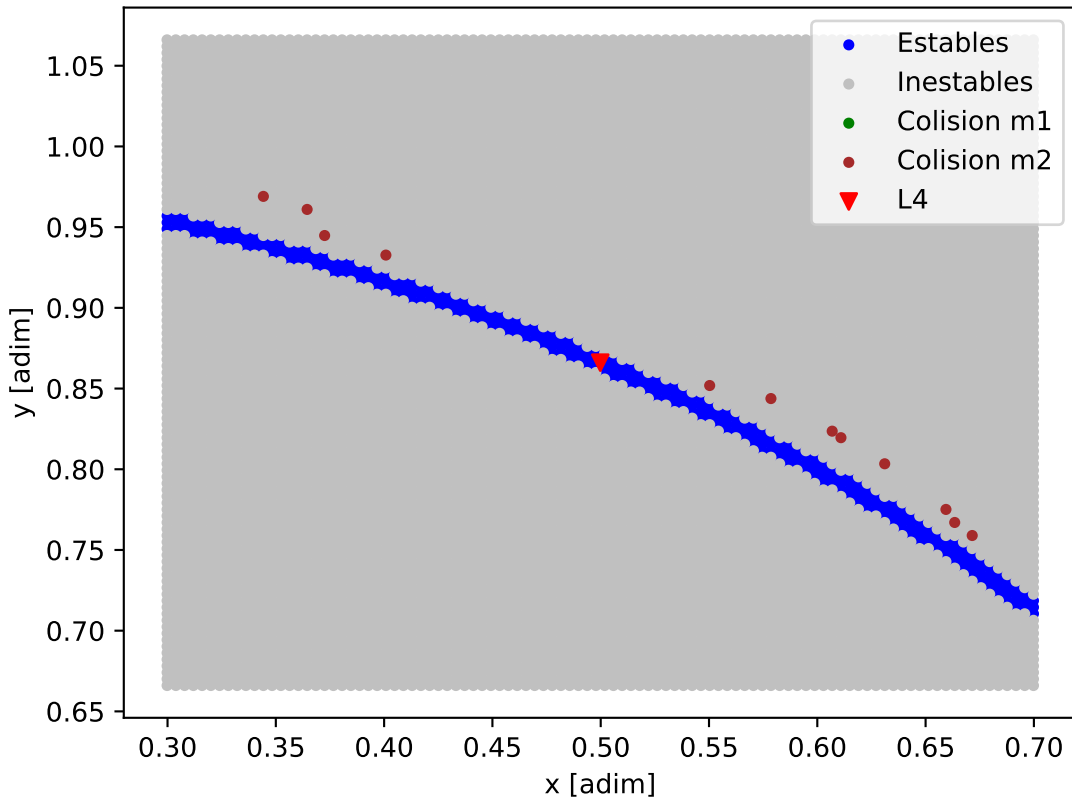
Mapa de estabilidad - DMPP-2
