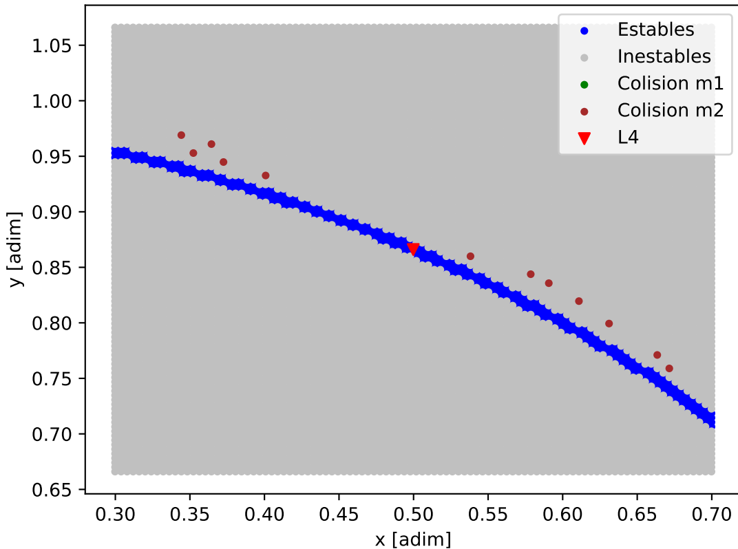
Mapa de estabilidad - HD_142
