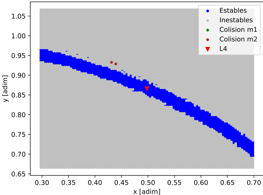
Mapa de estabilidad - HD_73344
