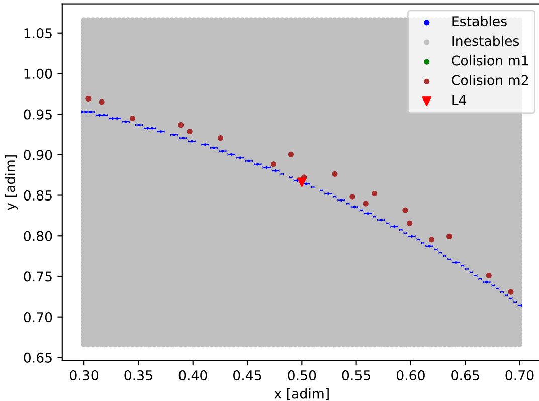
Mapa de estabilidad - TOI-201
