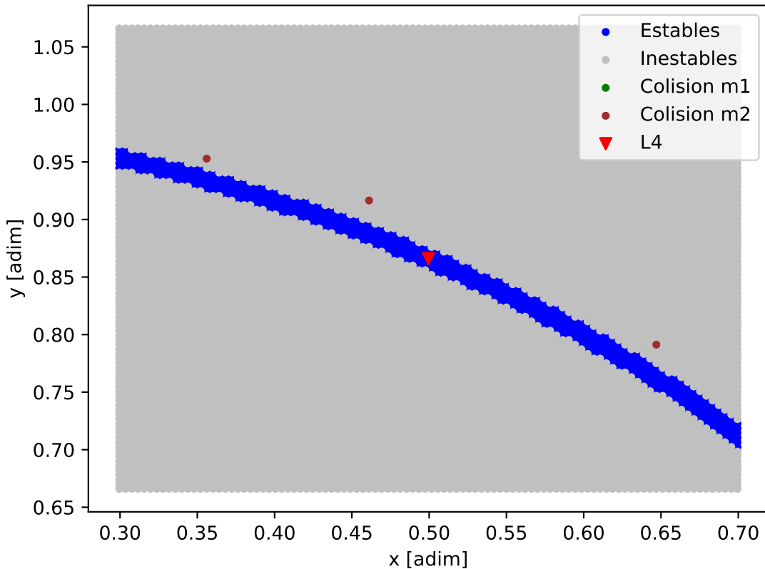
Mapa de estabilidad - ups_And
