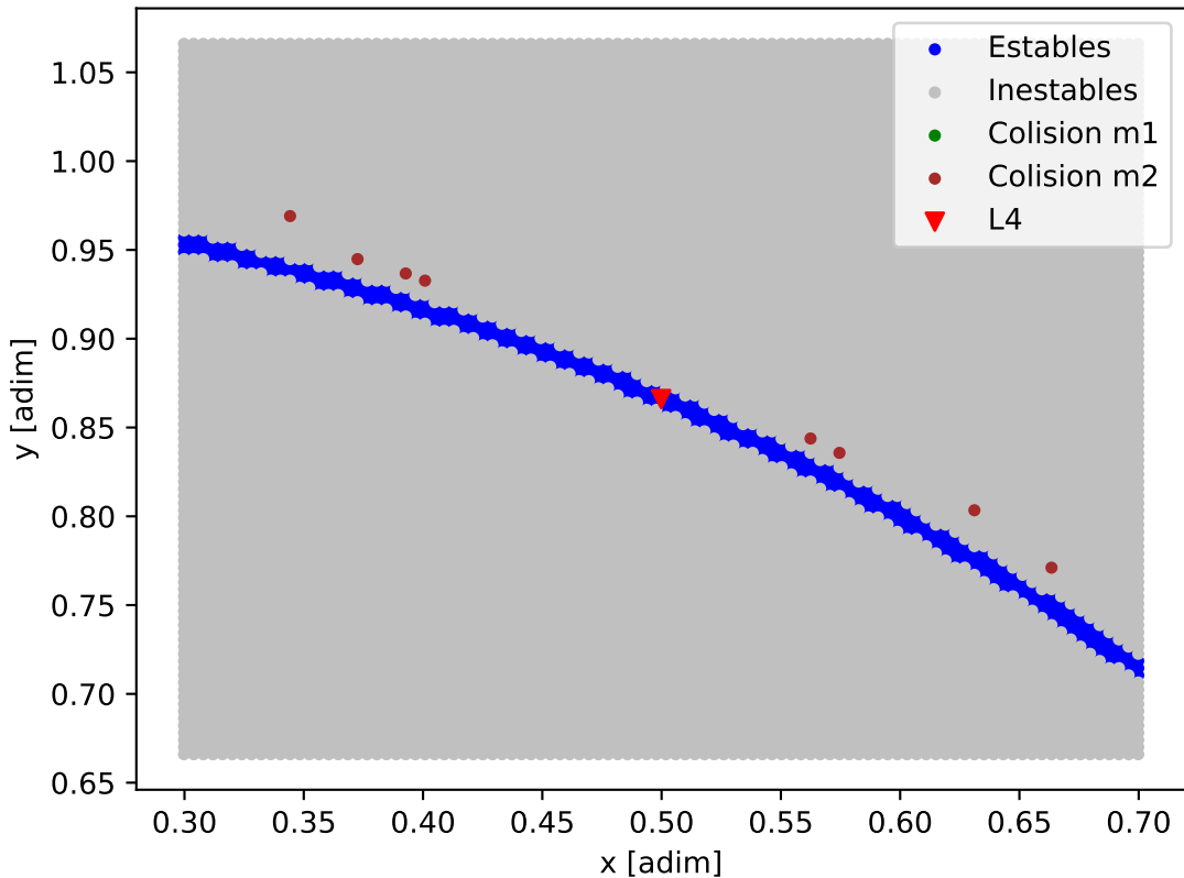
Mapa de estabilidad - HD_10180
