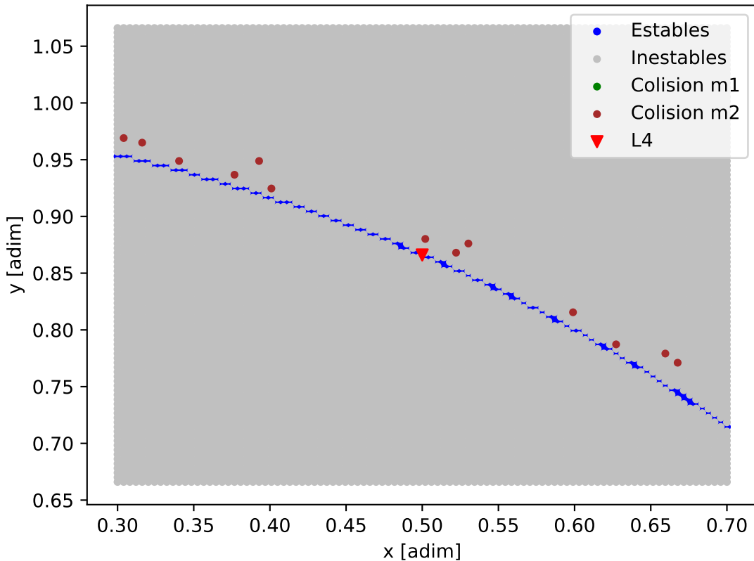
Mapa de estabilidad - HD_20794
