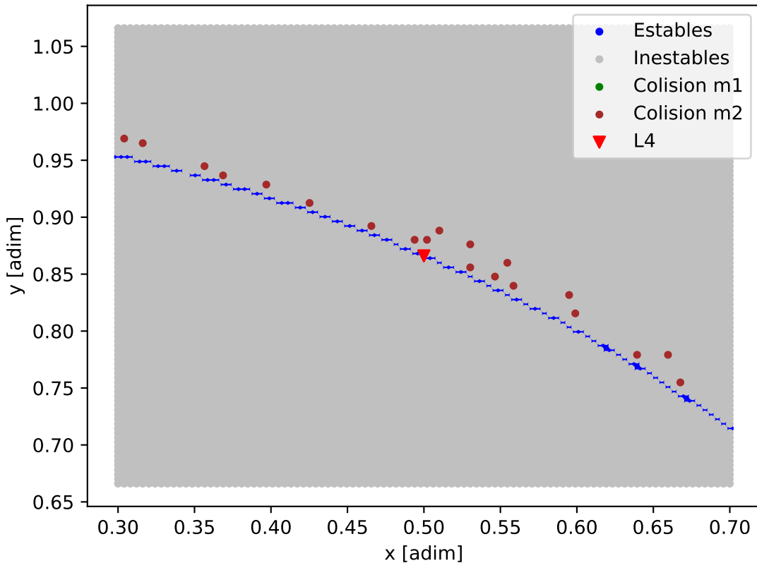
Mapa de estabilidad - HD_28471
